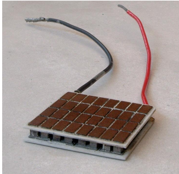
mein altes Modul mit einer Leistung von 20 Watt (Größe 3cm x3cm)
